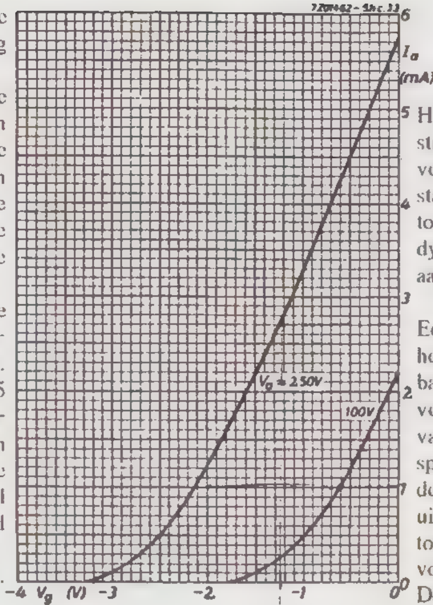
Figuur 12 ECC83 Ug-Ia karakteristiek
